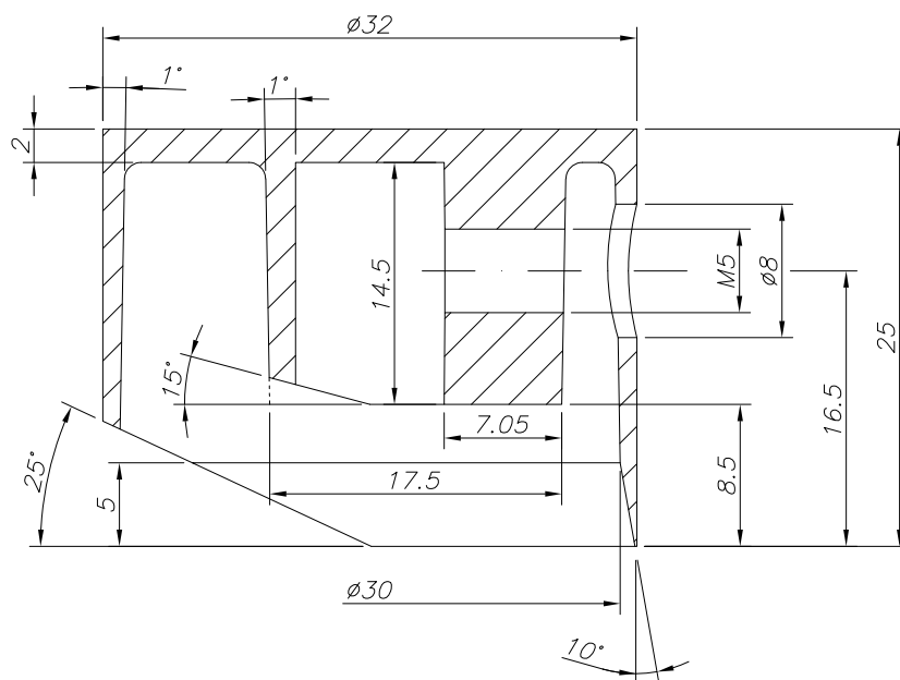
CORTE A-A
