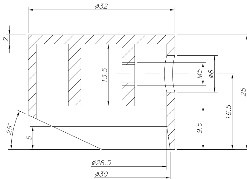
CORTE A-A
