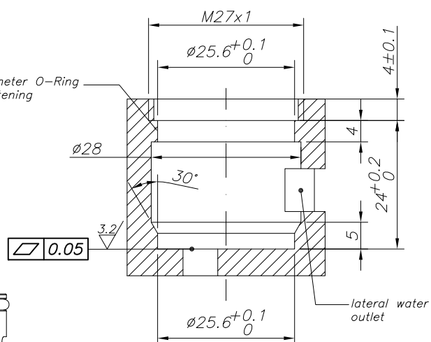
CORTE A-A
