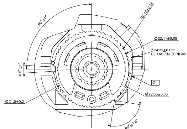
DETALLE B ESCALA 2/1 DENTADO RECTIL\NEO 60 DIENTES
