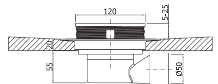
Sección desagüe horizontal
