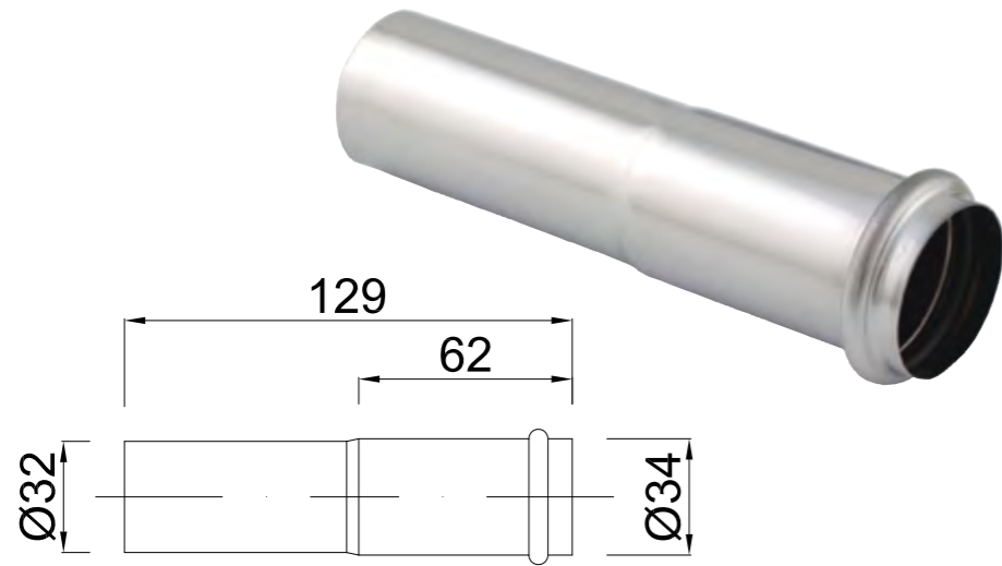
Tubo latón telescópico, Ø 32 mm x 130 mm Brass tube 32 Ø x 130 mm Tube Laiton Estensible Ø32 X 130 Mm
